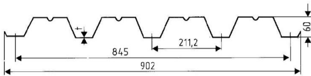
H60-845 ГОСТ 24045-94, ТУ 1122-079-02494680-01
