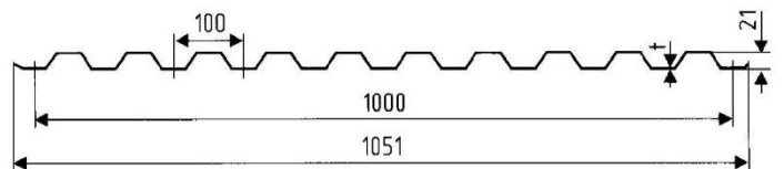
C21-1000 ГОСТ 24045-94, ТУ 1122-079-02494680-01
