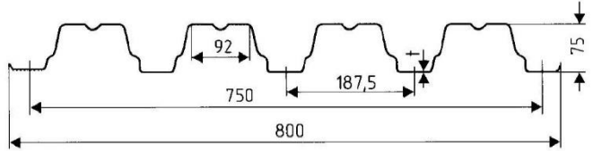
H75-750 ГОСТ 24045-94, ТУ 1122-079-02494680-01
