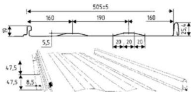
Фальцевая кровля "Классика"
