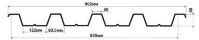
H60-845 ГОСТ 24045-94; ТУ 1122-079-02494680-01
